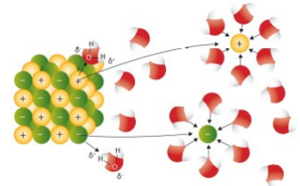
Solide ionique (à gauche) Ions en solution (à droite)
